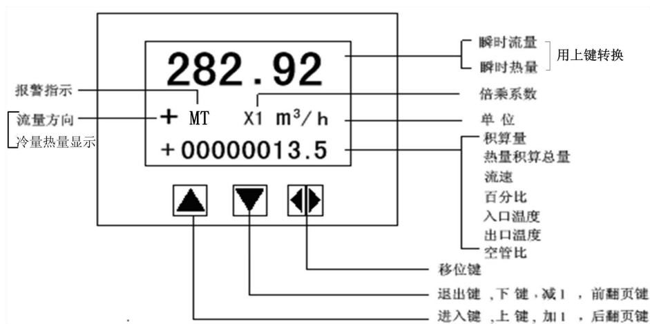
图 3.1 键盘定义与液晶显示
