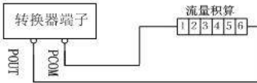
图 1.4 内供电接电子计数器
