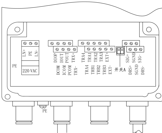
图 1.3 M8RBF22 主板接线端子图
