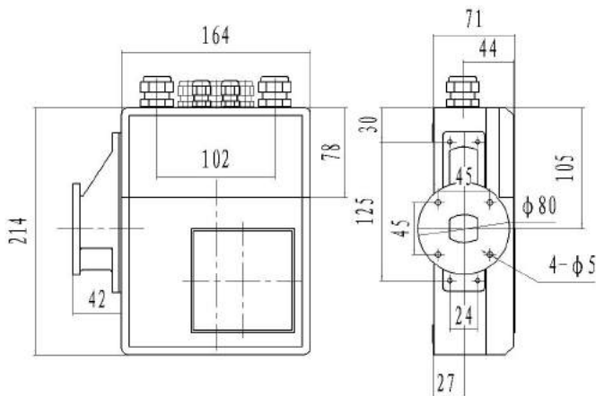
图 4.1 方型壳体分体式外型尺寸图
