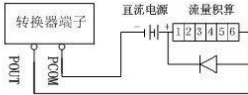
图 1.3 外供电接电子计数器
