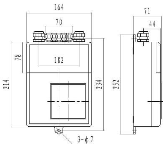
图 4.1 方型壳体分体式外型尺寸图
